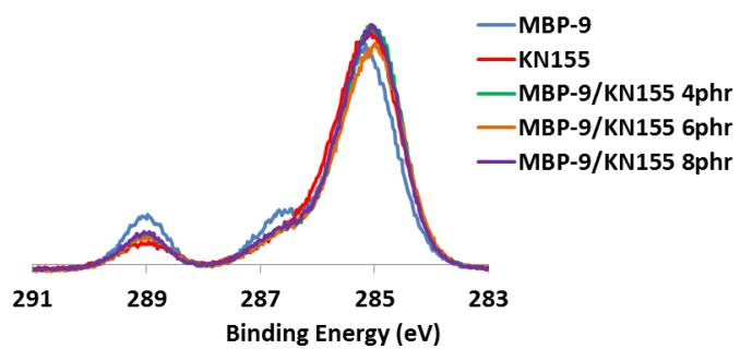
図 BP (MBP-9) に TF (KN155) を 4～8 部添加した粘着剤の XPS 測定による C1s スペクトル
